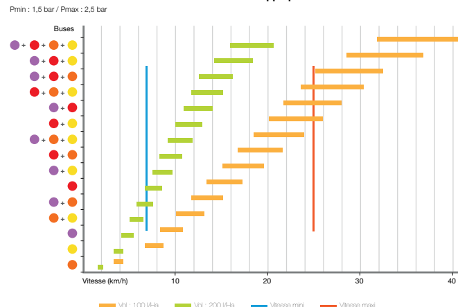
Sélection des buses selon la vitesse et/ou la dose appliquée
